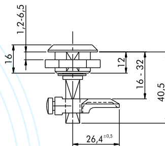
Montagem com lingueta curta
