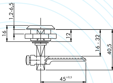
Montagem com lingueta longa
